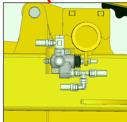
Capteur Hydraulique actif
