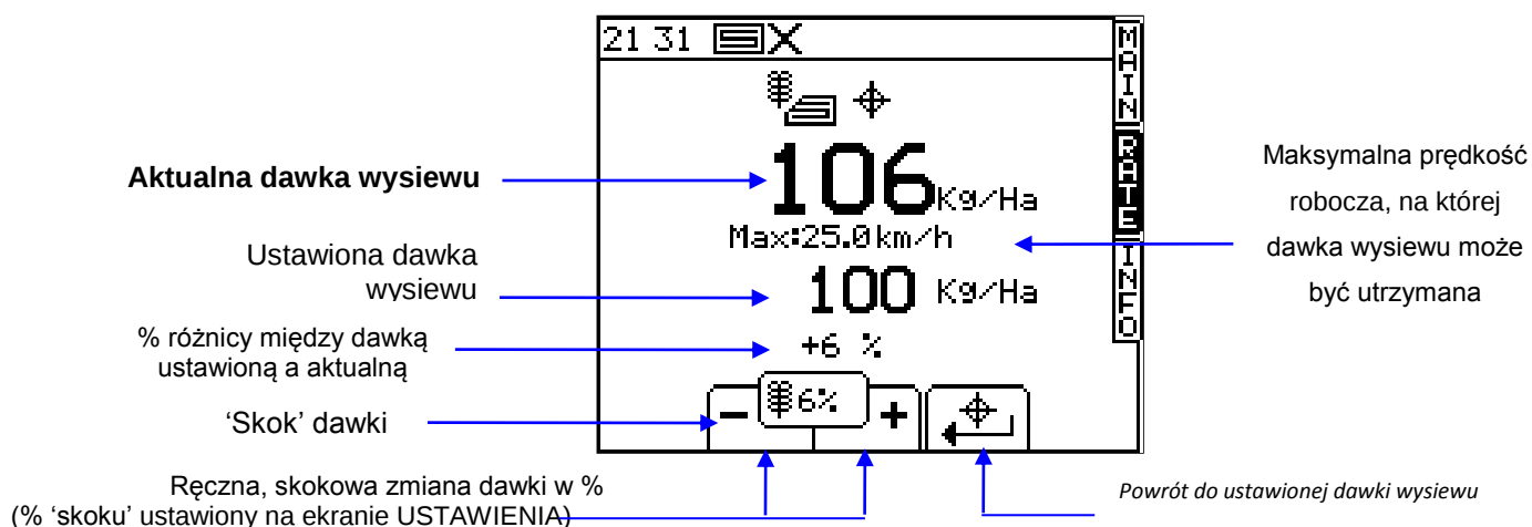
Figura 6: Ekran dawki wysiewu RATE – dozowanie jednego produktu
