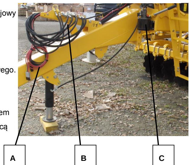
Figura 1 : Postój maszyny
