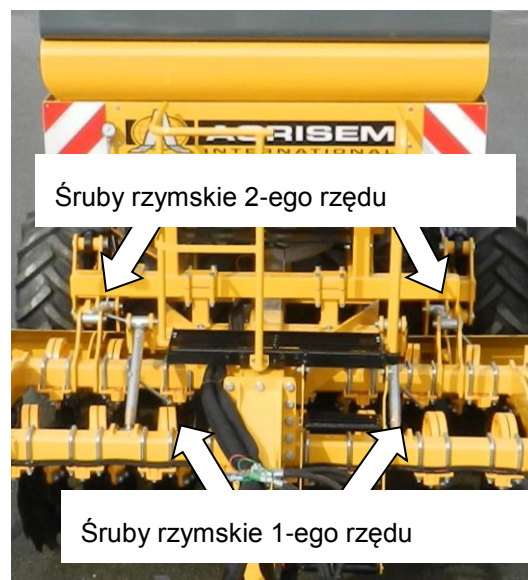
Figura 14 : śruby rzymskie (łączniki)
