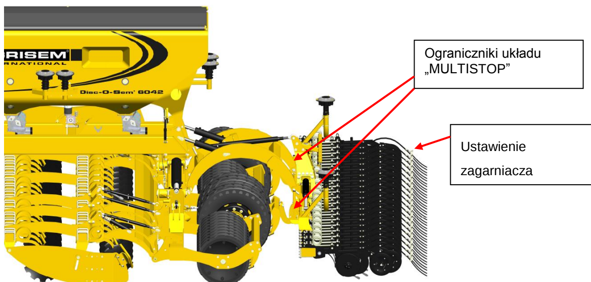
Figura 31 : Rozmieszczenie punktów regulacyjnych
