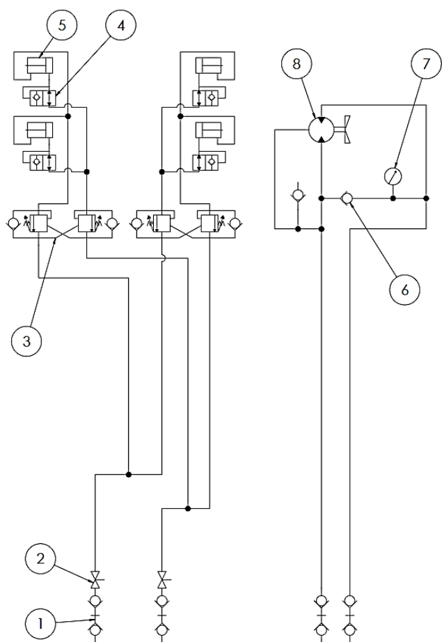
Circuito di chiusura e azionamento della turbina
