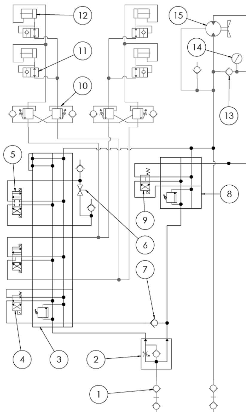
Circuito di chiusura e azionamento della turbina
